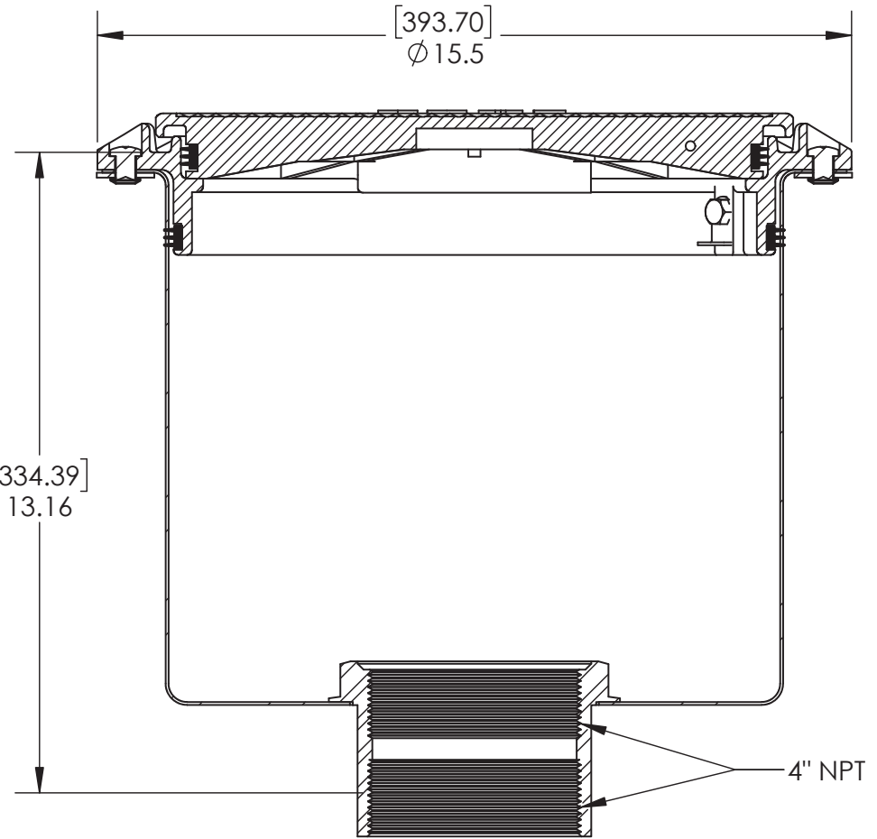
SECTION A-A SCALE 1 : 4
