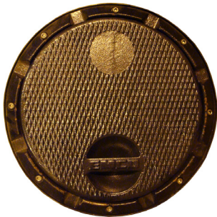
Rim 17.6"; Lid 15.3"
